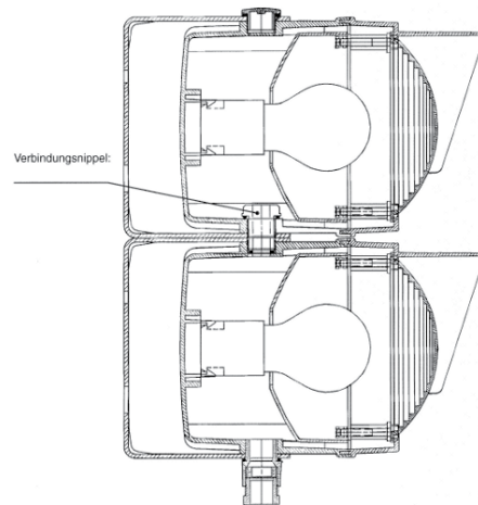
Schutzart IP65
