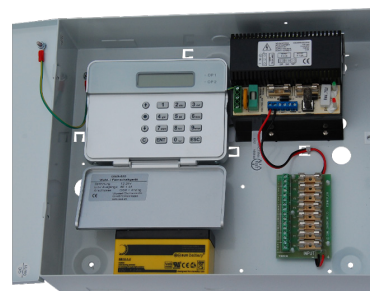
Klemmenfertiger Einbau in Notstromeinheit
